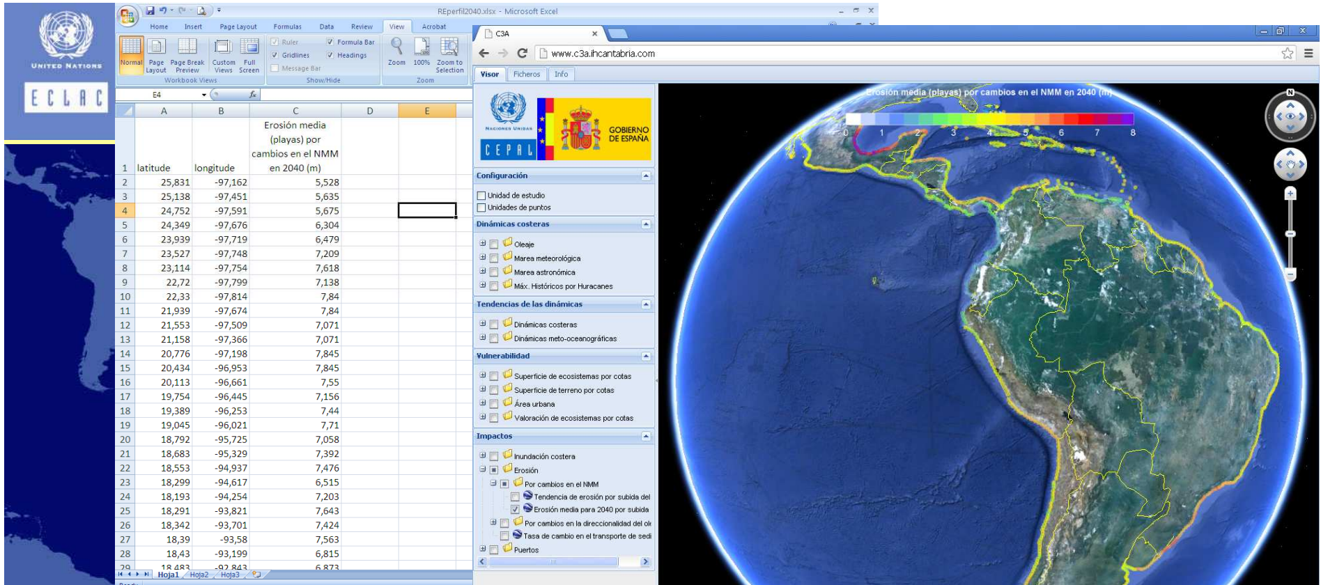
FIGURA 3.41 EROSIÓN DE LAS PLAYAS POR CAMBIOS EN EL PERFIL DE EQUILIBRIO EN 2040 (Metros)
